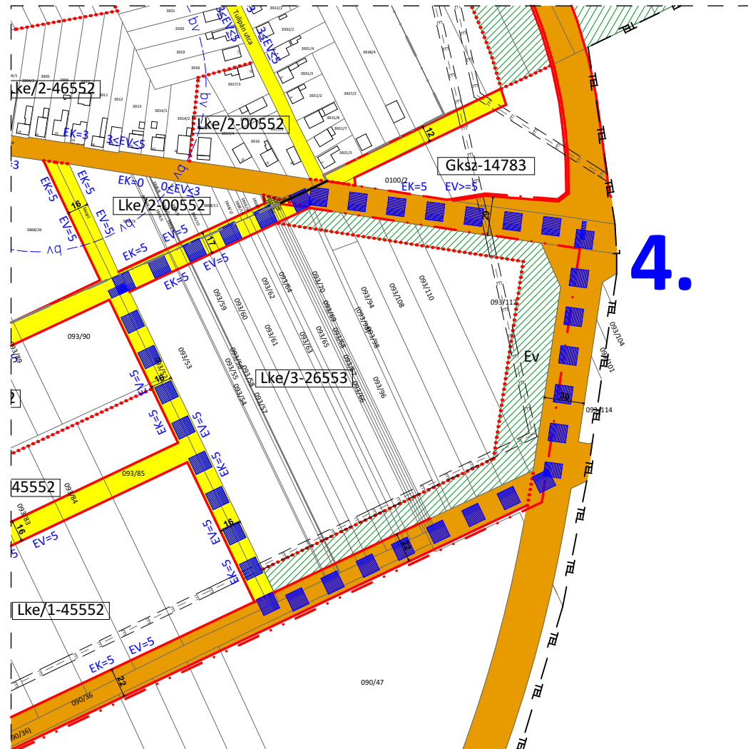
Hatályos terv részlete!
