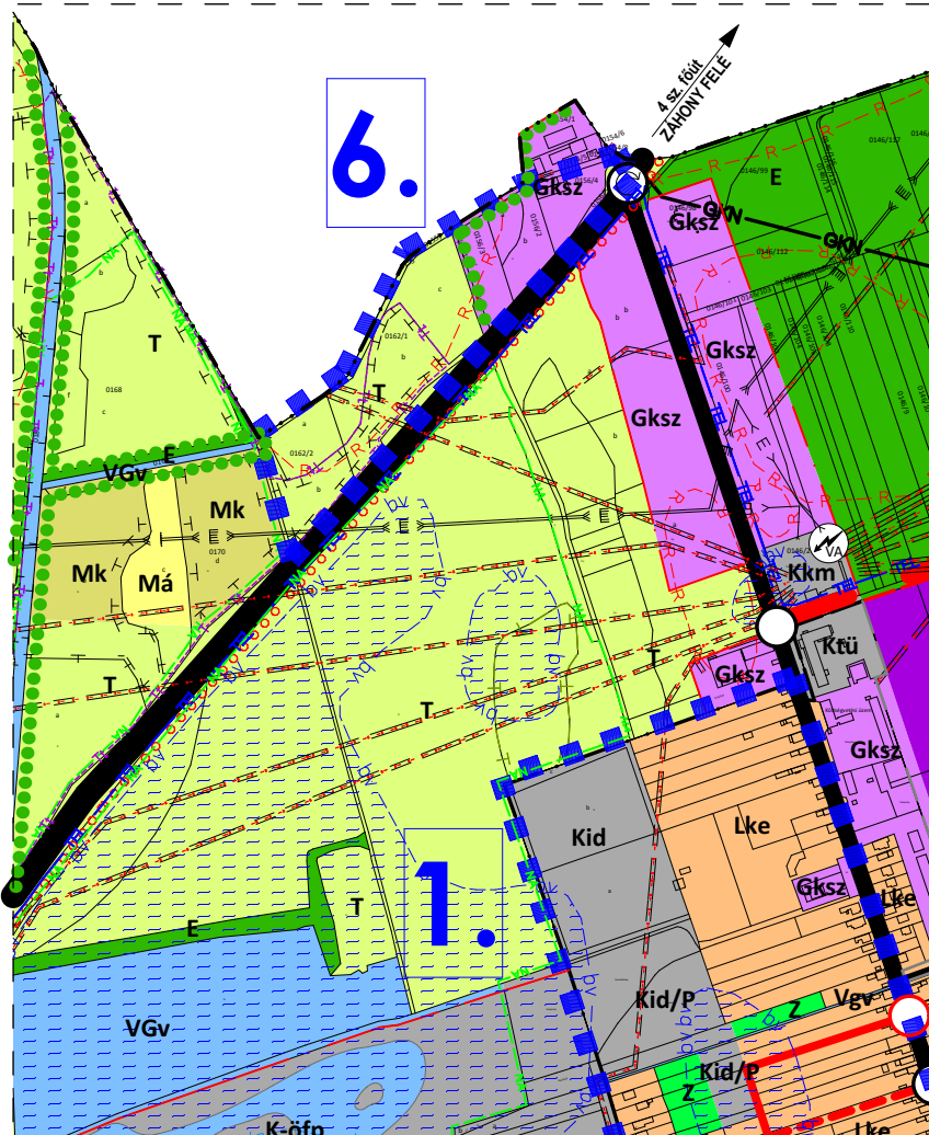
Hatályos terv részlete!
